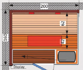
Design: KITZBÜHEL 160 Standard links Außenmaße: 200 x 160 x 200 cm (inkl. ca. 1 cm Hinterlüftung); Ofen Position kann getauscht werden (Türanschlag rechts); IR-Keramik- & Flächenstrahler sind optional Stand: 28.6.2019
