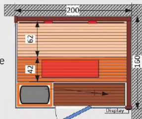
Design: KITZBÜHEL 160 Standard rechts Außenmaße: 200 x 160 x 200 cm (inkl. ca. 1 cm Hinterlüftung); Ofen Position kann getauscht werden (Türanschlag rechts); IR-Keramik- & Flächenstrahler sind optional
